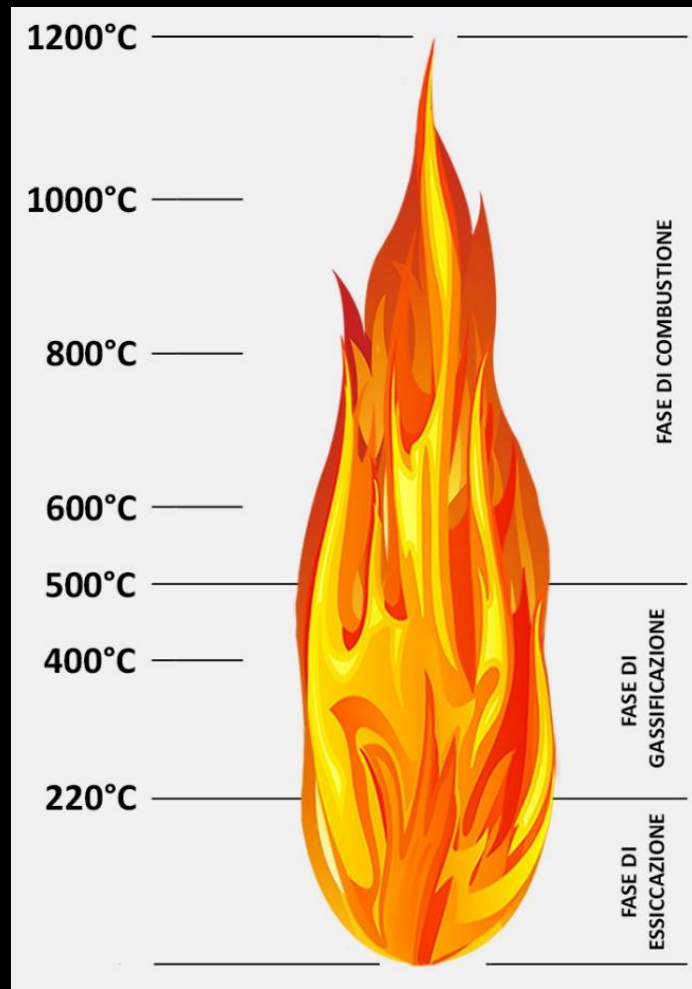
Temperatura all'interno della fiamma
