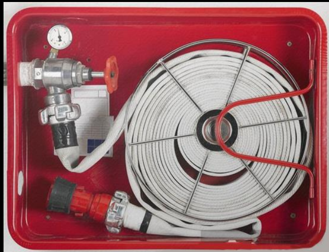
Impianti idrici fissi antincendio
