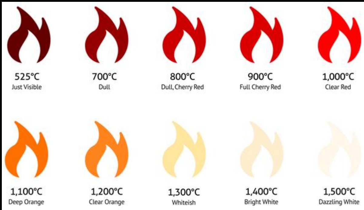
Colore della fiamma e sua temperatura
